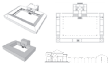
1. Desenhos de reconstrução da Vila Pisani.
